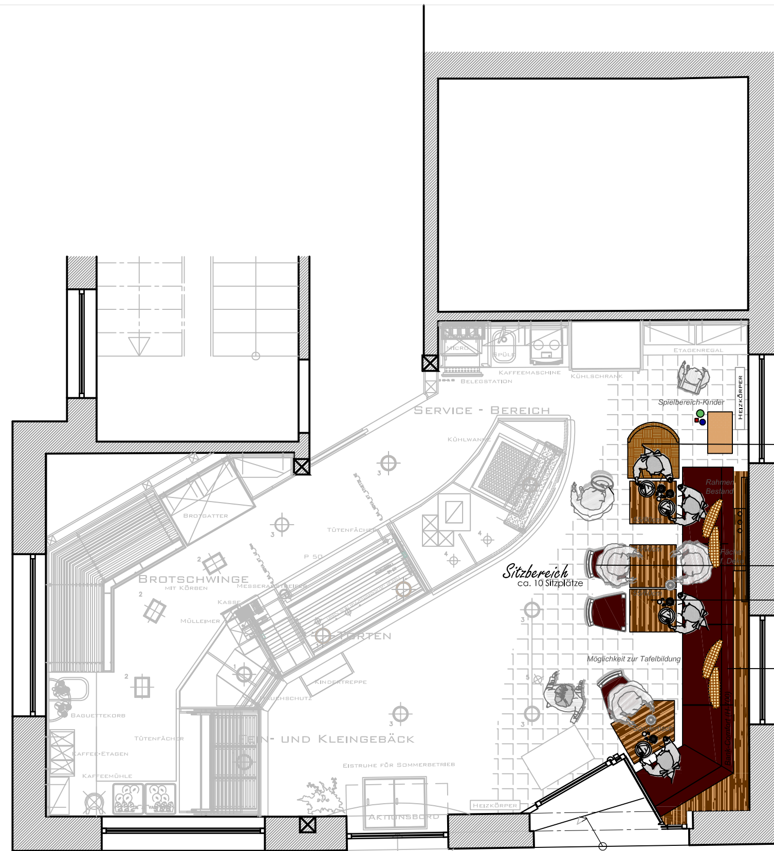
Grundriss
